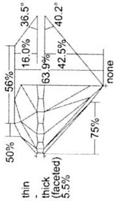
Profile to actual proportions
